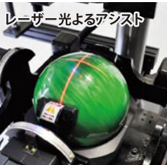
高精度LMガイドを使用。(X軸Y軸正確なドリルを補助します)
